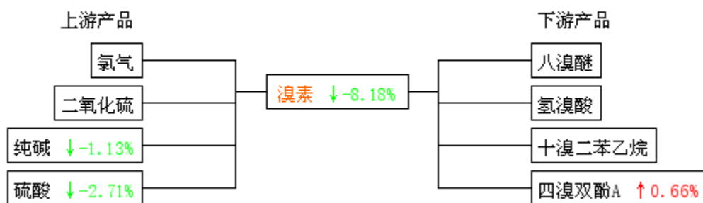
生意社溴素产业链价格涨跌图 2012-08-01 - 2012-08-31
