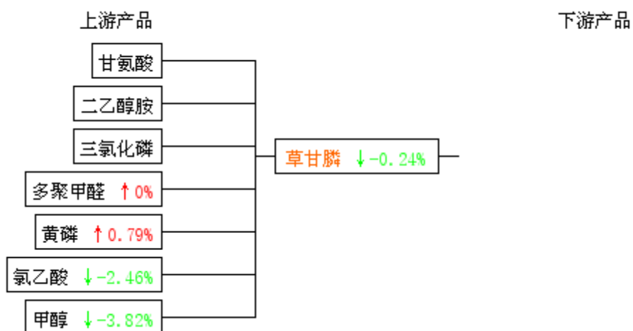
生意社草甘膦产业链价格涨跌图 2012-11-01 - 2012-11-30
