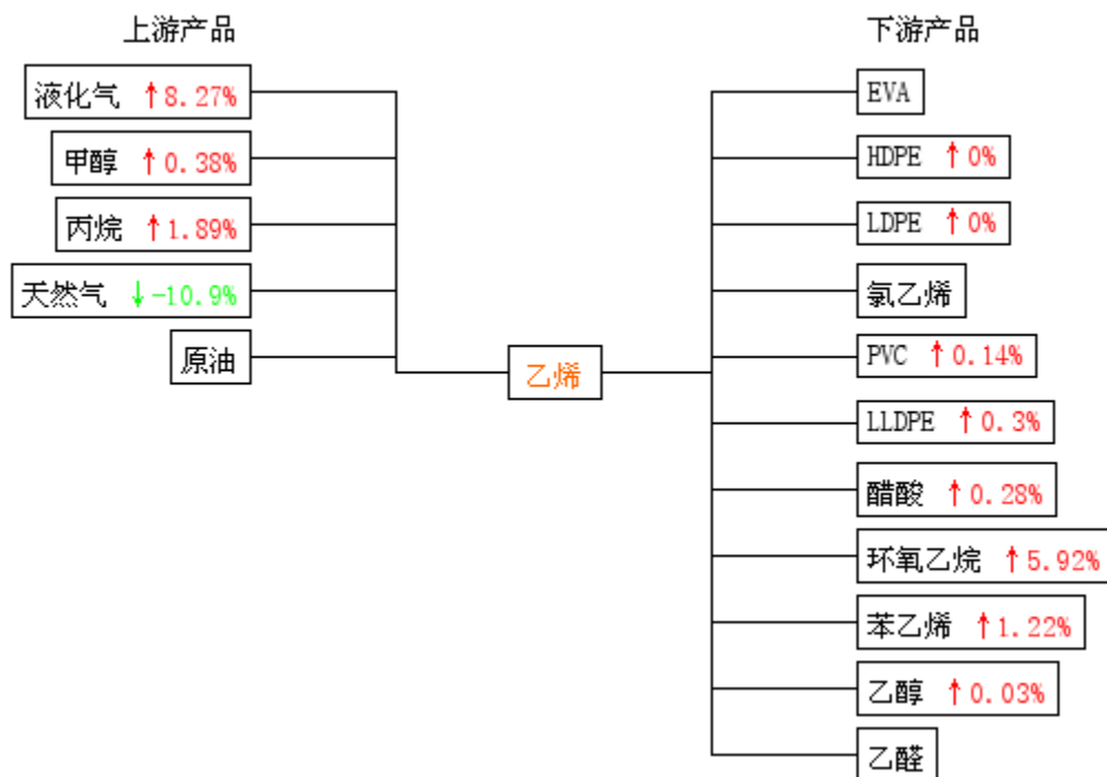
生意社乙烯产业链价格涨跌图 2013-02-01 - 2013-02-28
