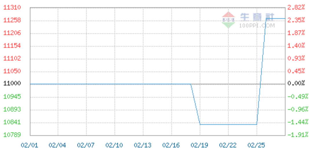
氧氯化锆 国内 生产者价格 2013-02-01 - 2013-02-28
