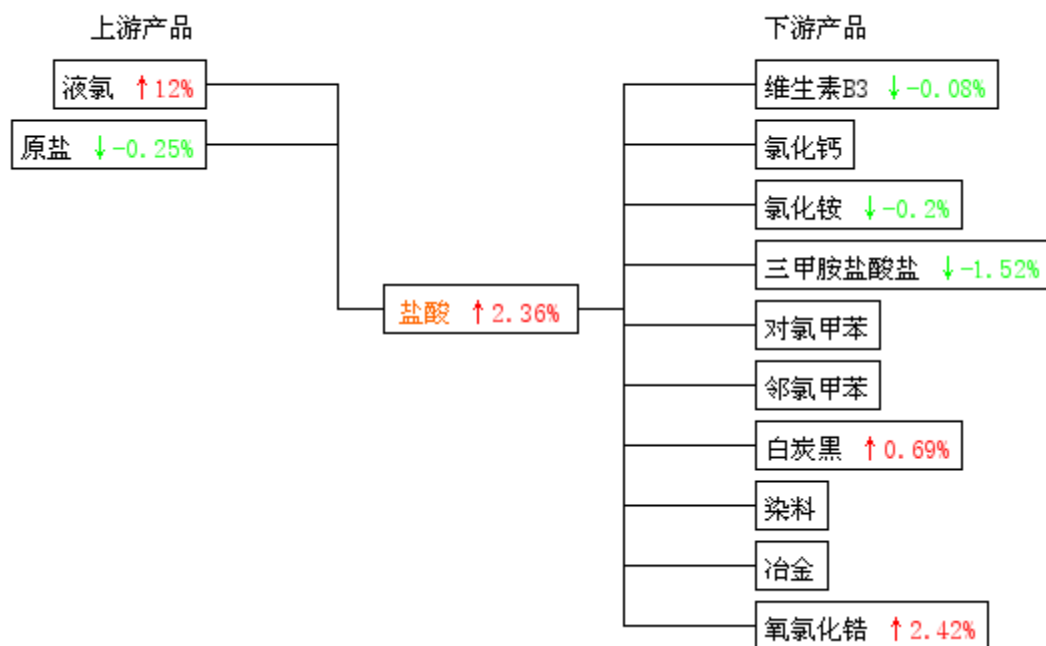
生意社盐酸产业链价格涨跌图 2013-02-01 - 2013-02-28
