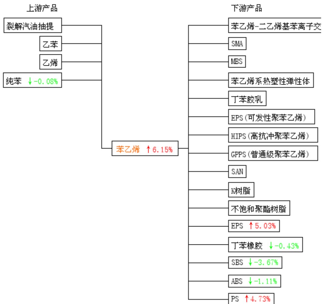
生意社苯乙烯产业链价格涨跌图 2013-07-01 - 2013-07-31
