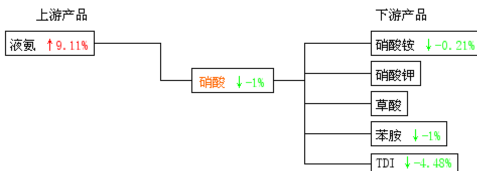
生意社硝酸产业链价格涨跌图 2013-11-01 - 2013-11-30
