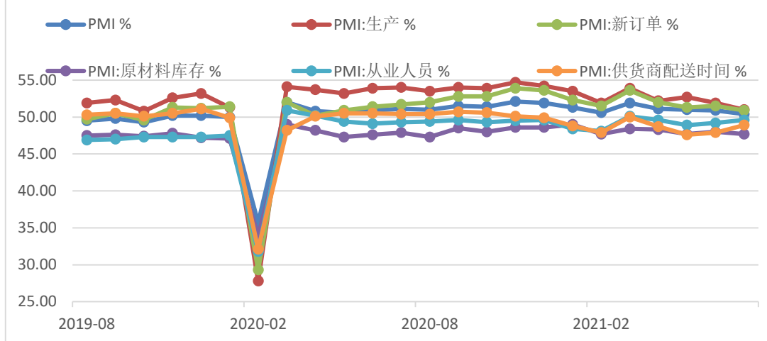
图9.PMI指数
