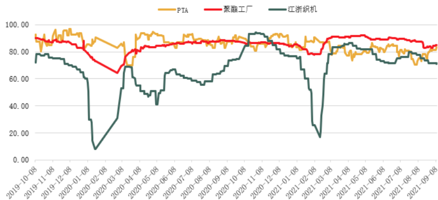
图 2:PTA 产业链开工率
